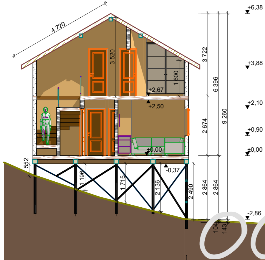
Разрез 1-1
